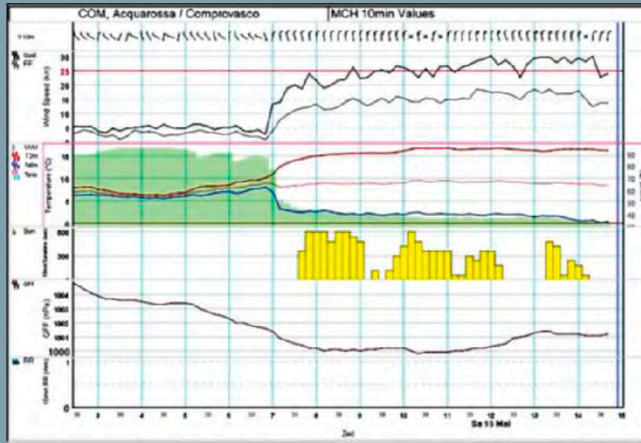
Die Messwerte der Wetterstation von Comprovasco im Tessin zeigen einen typischen Durchbruch des Nordföhns. Schon morgens früh steigen die Windgeschwindigkeiten talauswärts sprunghaft an. Bei vorhandener Bodeninversion kann sich der Durchbruch verzögern. Wer dann schon in der Luft ist, bekommt bei der Landung Probleme.
