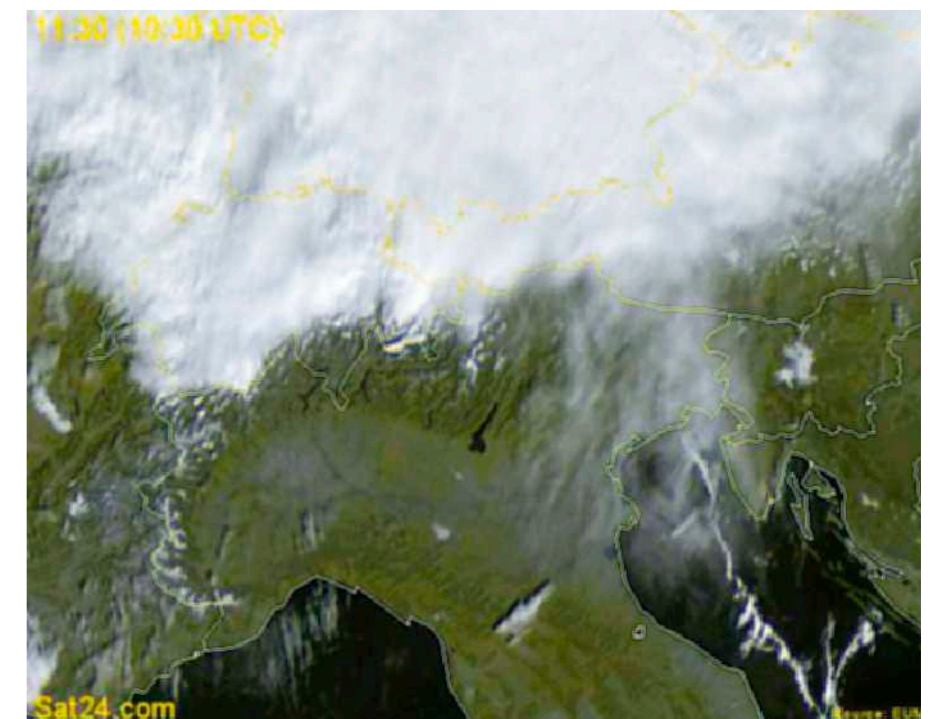
Eine typische Nordföhnsituation im Satellitenbild. Die kalte Luft staut sich in den Nordalpen, gut sichtbar an der dichten Wolkendecke. Südlich des Alpenhauptkamms ist es dagegen klar. Die Sonne kann ungehindert einstrahlen. Das sorgt für gute Thermik, bei durchgreifendem Nordwind aber auch für gefährliche Turbulenzen.
