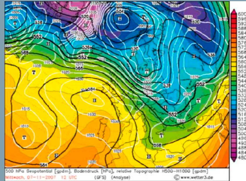
Eine typische Nordföhnlage. Nach dem Durchzug eines Tiefs samt Kaltfront rückt von Westen her ein Hoch nach. Die weiß eingezeichneten Isobaren des Boden-
