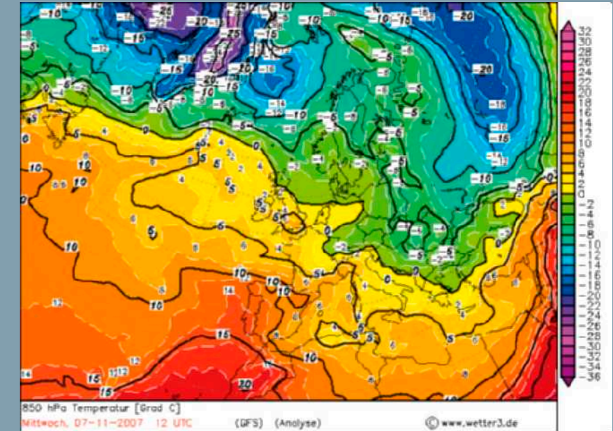
Die prognostizierte Lufttemperatur in 1.500 Meter Höhe ist ein guter Indikator für riskante Nordföhnlagen. Je größer die Temperaturunterschiede nördlich und südlich der Alpen, desto eher greift der Nordföhn weit in die südlichen Täler durch.
