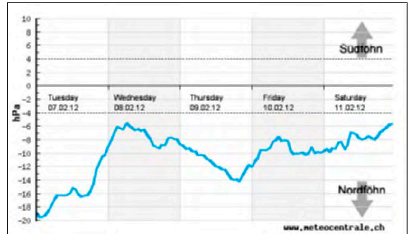
Ein Diagramm der Druckdifferenzen zwischen Nord- und Südalpen (Zürich und Lugano). Je größer der Unterschied, desto höher ist die Wahrscheinlichkeit, dass Föhn auftritt. Solche Grafiken gibt es unter www.meteocentrale.ch/de/wetter/foehn-und-bise/foehn.html .
